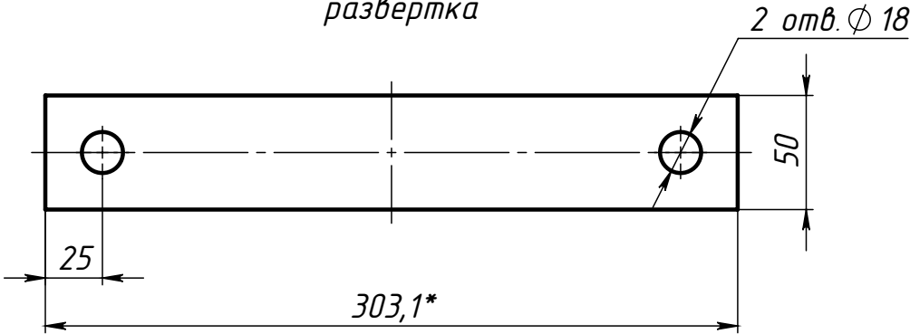
Поз.4 (Полухомут) развертка
