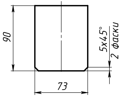
Поз.3 (Ребро среднее)
